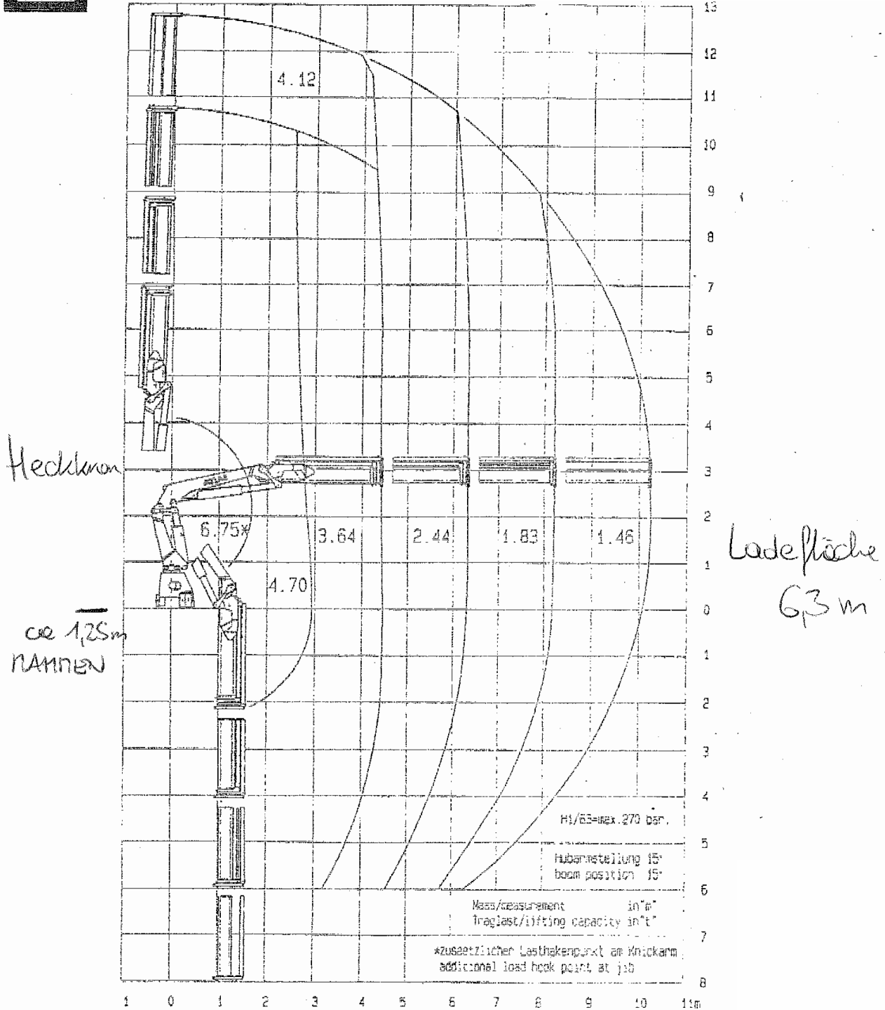
(A3) ATLAS 170.1-10.3/3 Traglastdiagramm Load diagram 4205.000.00.00 / 022
